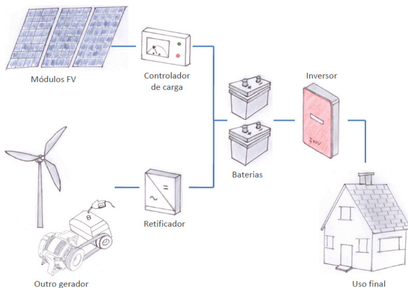
Figura 2.9 - Sistema híbrido.
