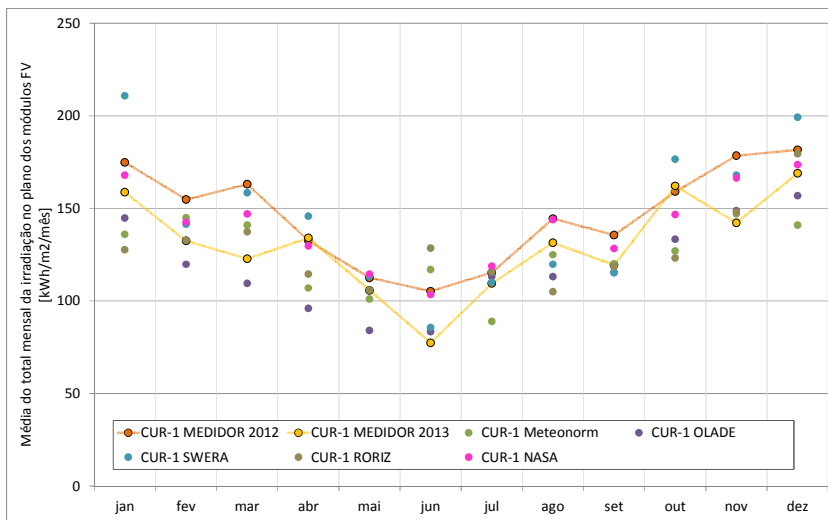
Figura 0.24 - CUR-1: Média do total mensal da irradiação no plano dos módulos FV (kWh/m²/mês)
