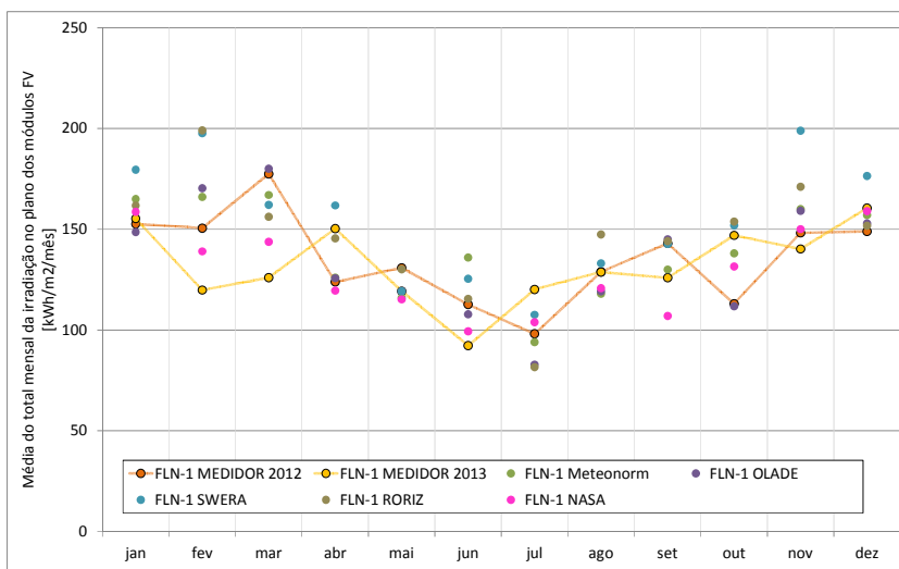
Figura 5.9 - SFVCR FLN-1: Média do total mensal da irradiação no plano dos módulos FV (kWh/m²/mês)
