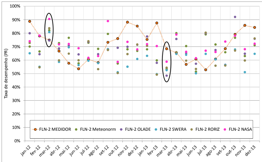
Figura 0.2 - FLN-2: PR ao longo de dois anos medidos (2012-2013) X PR referente a banco dedados.
