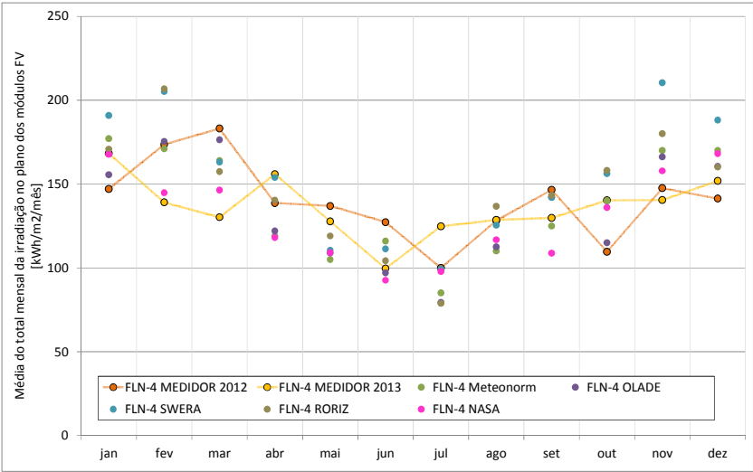
Figura 0.7 - FLN-4: Média do total mensal da irradiação no plano dos módulos FV (kWh/m²/mês)
