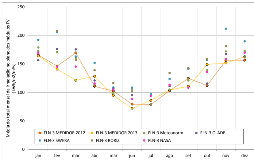
Figura 0.4 - FLN-3: Média do total mensal da irradiação no plano dos módulos FV (kWh/m²/mês)
