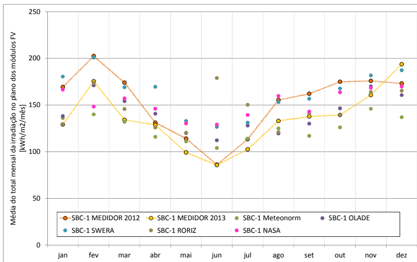
Figura 0.18 - SBC-1: Média do total mensal da irradiação no plano dos módulos FV (kWh/m²/mês)
