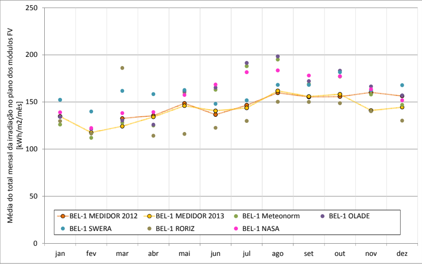
Figura 0.27 - BEL-1: Média do total mensal da irradiação no plano dos módulos FV (kWh/m²/mês)
