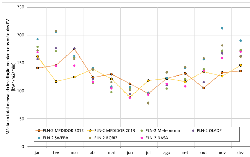
Figura 0.1 - FLN-2: Média do total mensais da irradiação no plano dos módulos FV (kWh/m²/mês)
