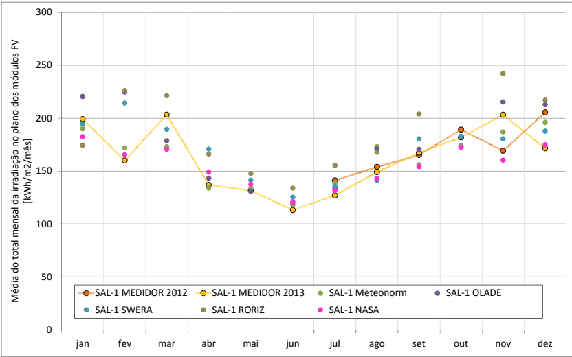
Figura 0.13 -SAL-1: Média do total mensal da irradiação no plano dos módulos FV (kWh/m²/mês)
