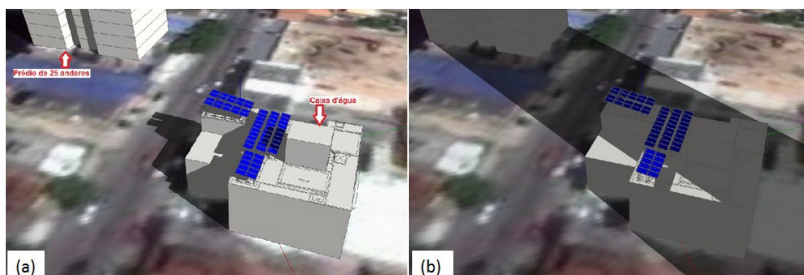
Figura 3.14 - BEL 1: Projeções de sombra no SFVCR nos dias e horários de (a) 21 de junho às 9 h e (b) 21 de dezembro às 16 h.
