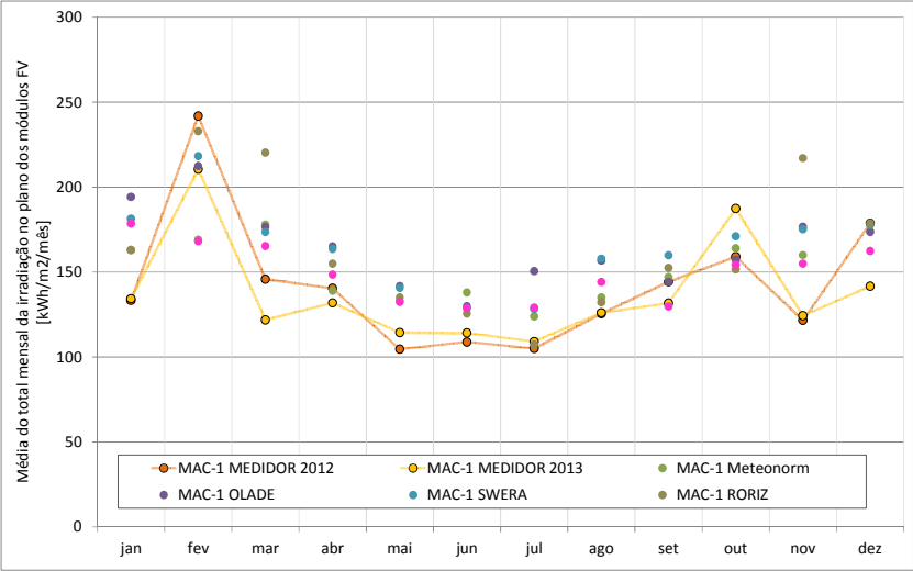
Figura 0.21 - MAC-1: Média do total mensal da irradiação no plano dos módulos FV (kWh/m²/mês)
