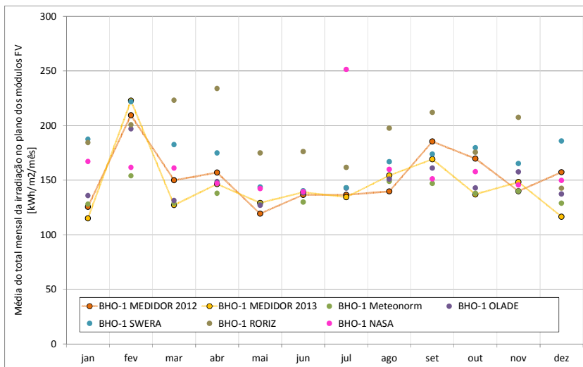
Figura 0.10 -BHO-1: Média do total mensal da irradiação no plano dos módulos FV (kWh/m²/mês)
