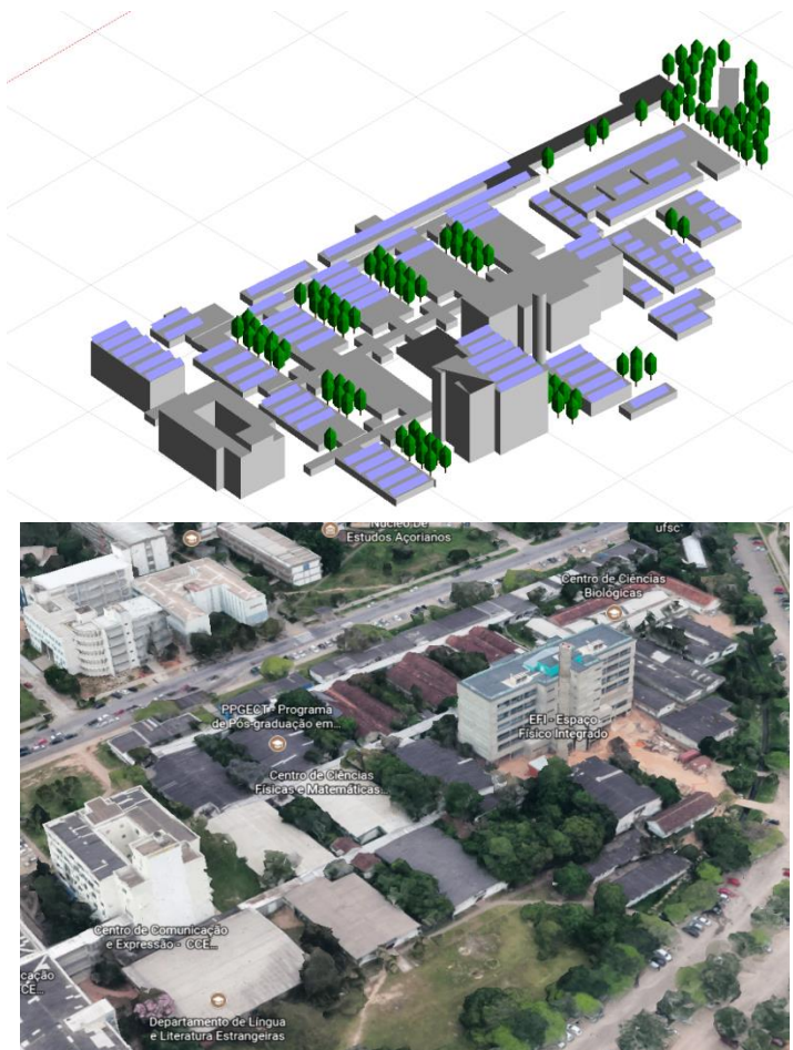
Figura 19 – Modelagem 3D da instalação solar fotovoltaica do CFM-CCB-EFI. Fonte: Adaptado sobre imagem do Google Earth.
