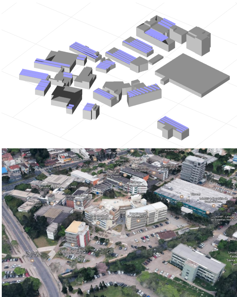
Figura 20 – Edificações selecionadas para Centro Tecnológico da UFSC em Florianópolis-SC, com a localização das respectivas instalações solares fotovoltaicas.
