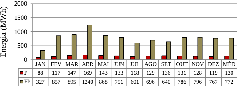
Figura 42– Evolução mensal da energia ativa consumida na UC Cidade Universitária – UFSC em Florianópolis-SC, considerando a operação de uma usina solar fotovoltaica de 5 MW instalada no Campus Central da UFSC em 2016.
