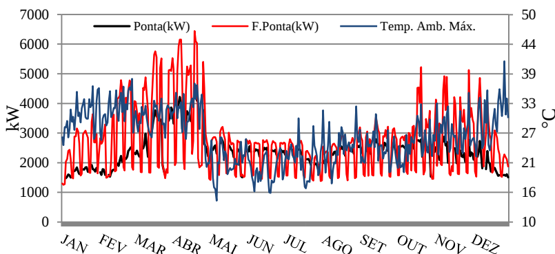
Figura 23 – Demandas medidas nos horários P e FP e temperaturas ambientes máximas registradas na UC Cidade Universitária UFSC em Florianópolis-SC.
