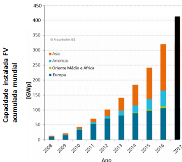
Figura 1 – Evolução da capacidade instalada FV acumulada.
