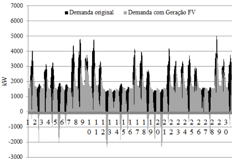
Figura 75 - Evolução diária de demanda original e da demanda com a contribuição de minigeração FV de 5 MW - Novembro.
